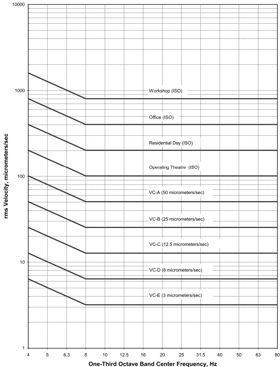
Bild A.1 VC-Kriterien nach Gordon
