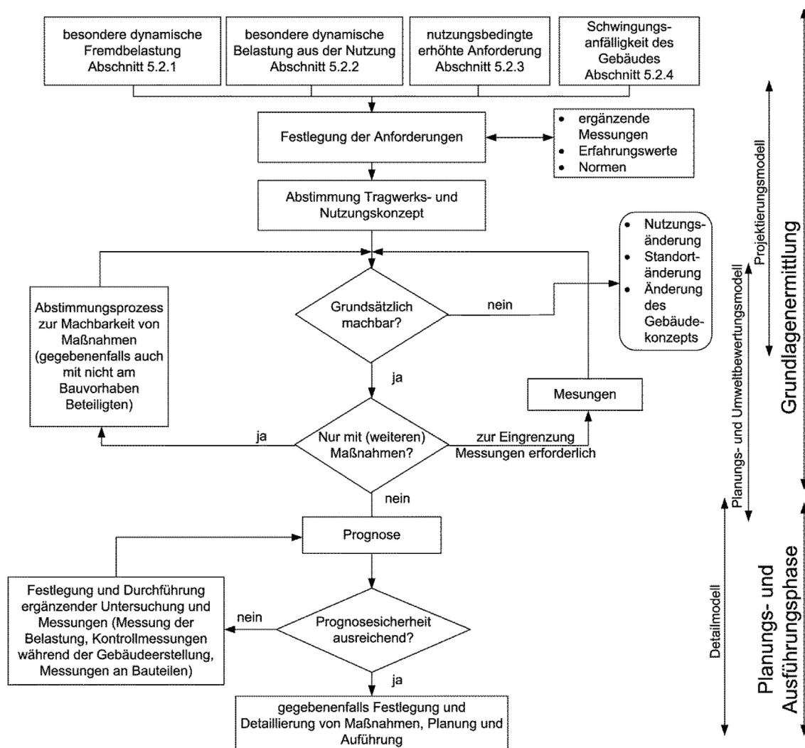
Bild 2.1 Ablauf einer baudynamischen Planung (aus VDI 2038, Blatt 1, Bild 3)
