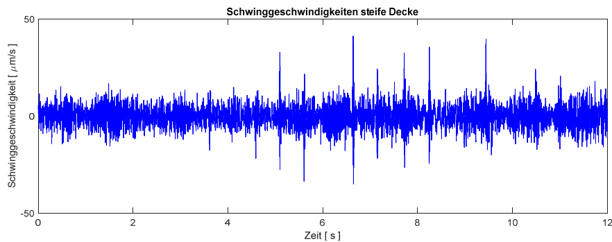
Bild 4.5 Schwinggeschwindigkeiten einer steifen Decke (Eigenfrequenz > 25 Hz), wenn eine Person 2 Meter neben dem Sensor vorbei geht.
