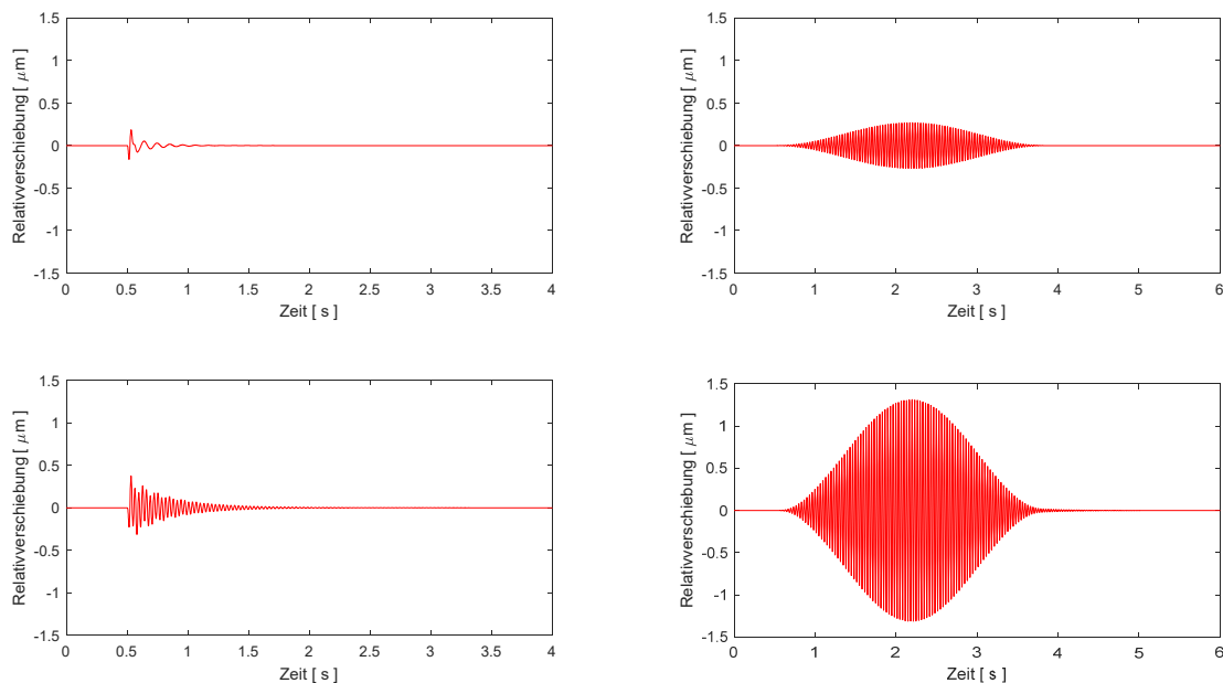
Bild 3.4 Relativverschiebung zwischen Objektiv und Objekt links für den kurzen und rechts für den langen Puls - oben jeweils für eine hohe interne Dämpfung und unten für ein schwach gedämpftes System.
