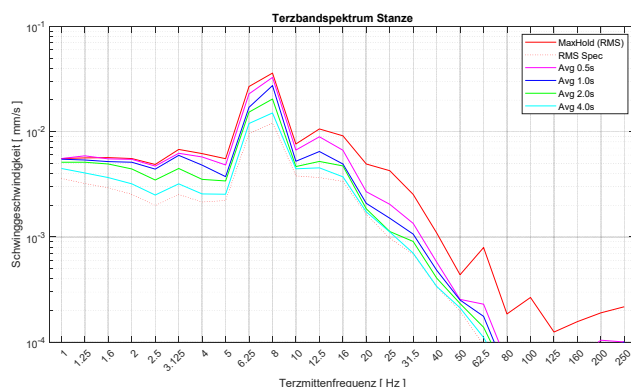
Bild 4.4 Terzbandspektren des in Bild 4.3 gezeigten Signales mit unterschiedlichen Mittelungszeiten.
