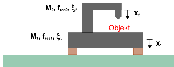
Bild 3.2 Vereinfachtes System, als Zweimassenschwinger idealisiert.
