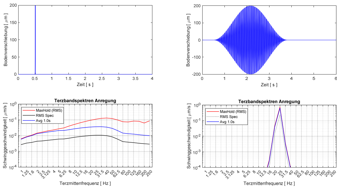
Bild 3.3 Anregung des Systems mit kurzem Puls (links) und mit langen Puls mit definierter Hauptfrequenz (rechts) und die zugehörigen Terzbandspektren.
