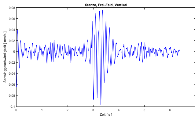
Bild 4.3 Vertikale Erschütterungen infolge einer Stanze in ca. 100 m Entfernung, gemessen im freien Feld.
