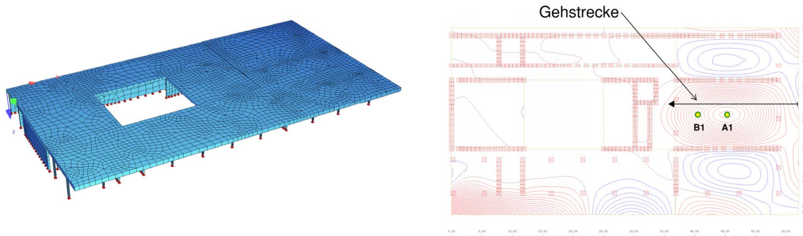
Bild 5.1 Ausschnitt aus dem Simulationsmodell (links). Simulationsmodell mit Gehstrecke, Messpunkten und hinterlegtem ersten Schwingungsmod bei 16 Hz (rechts).
