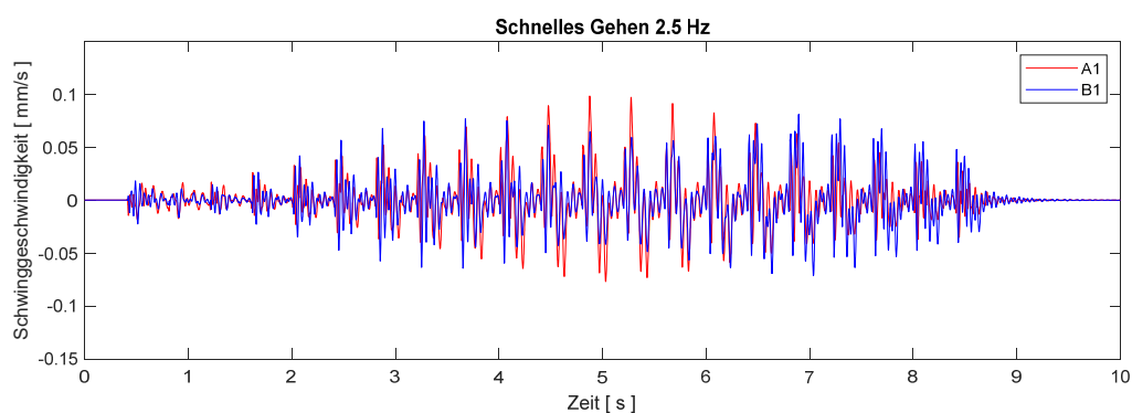
Bild 5.2 Numerisch ermittelte Schwinggeschwindigkeiten an den Punkten A1 und B1 während eine Person mit 2.5 Hz (= Schritte/Sekunde) relativ schnell neben den Messpunkten vorbei geht.
