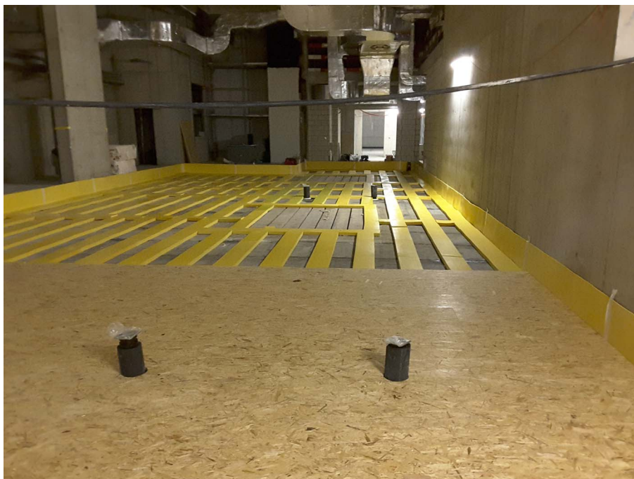
Bild 6.1 Bauzustand einer elastisch gelagerte Sockelplatte aus Beton im Bereich der Haustechnikanlagen.
