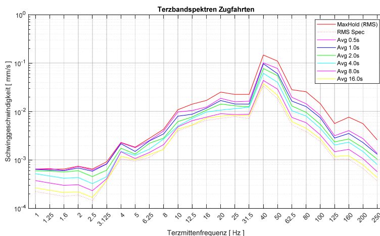
Bild 4.2 Terzbandspektren des in Bild 4.1 gezeigten Signales mit unterschiedlichen Mittelungszeiten.
