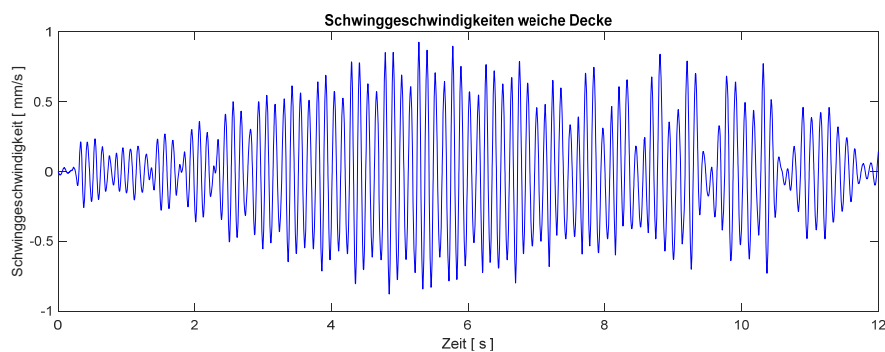
Bild 4.6 Schwinggeschwindigkeiten einer weichen Decke (8.1 Hz Eigenfrequenz), wenn eine Person 1 Meter neben dem Sensor vorbei geht.
