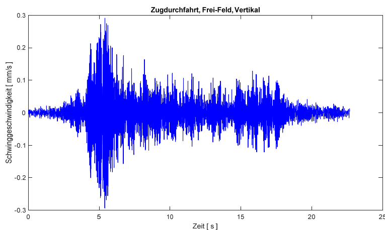
Bild 4.1 Vertikale Erschütterungen einer Zugdurchfahrt, gemessen im freien Feld.
