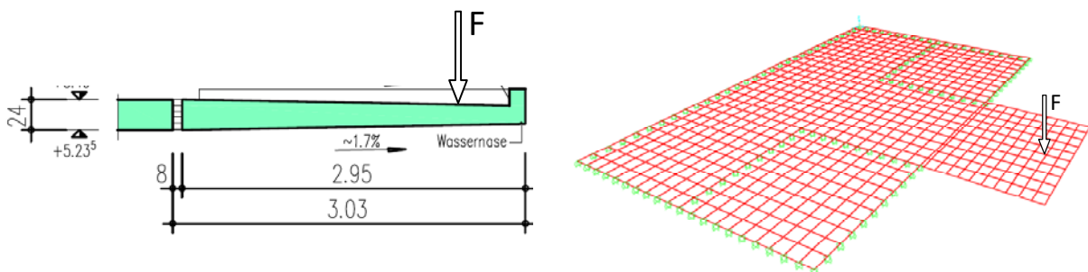
Bild 4.1 Querschnitt und FE-Modell
